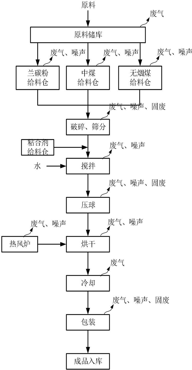
图 3-5 生产工艺流程图及产排污环节
